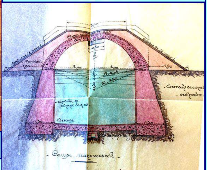
Ci-dessus : Plan des filtres à l'entrée du réservoir fait à la main en 1909
