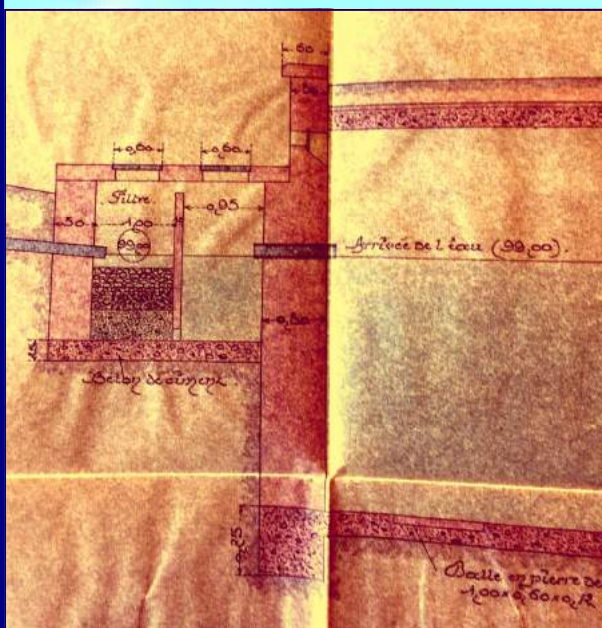
Ci-dessus : Plan des filtres à l'entrée du réservoir fait à la main en 1909
